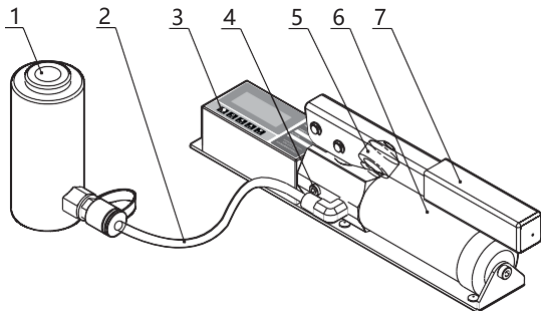
1. 液压缸 2. 高压油管 3. 数显压力表 4. 注油孔 5. 卸荷阀 6. 储油筒 7. 压杆
